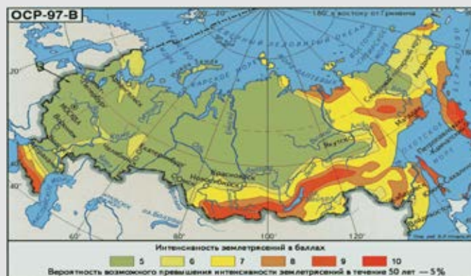
На изображении показаны зоны сейсмической активности России
