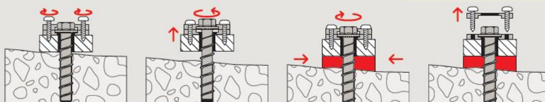
Необязательное удаление шайбы FSW
