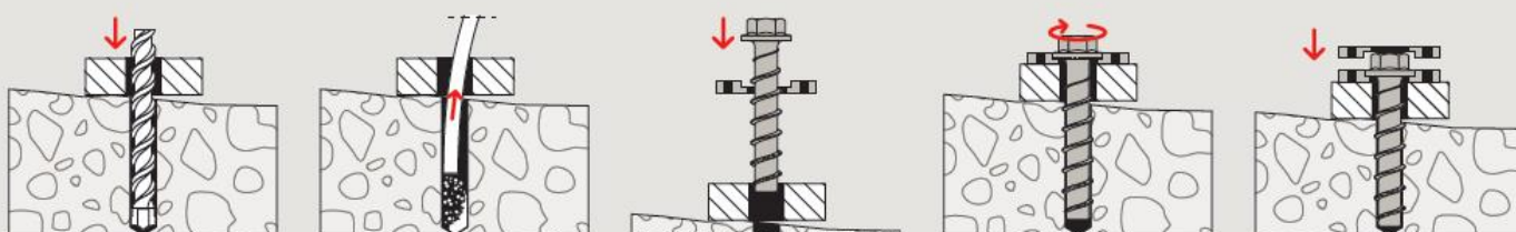
Необязательное удаление шайбы FSW
