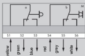
Схема підключення допоміжних контактів NAFA...20S
