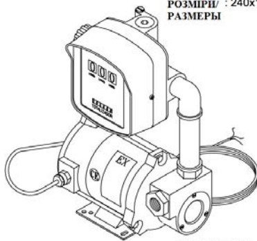
SAG-500 EExd ВАГА/ВЕС: 13Kg РОЗМІРИ/ 240x165x335mm РАЗМЕРЫ
