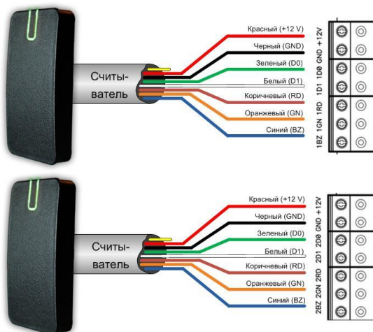
Рис.11. Подключение считывателей
