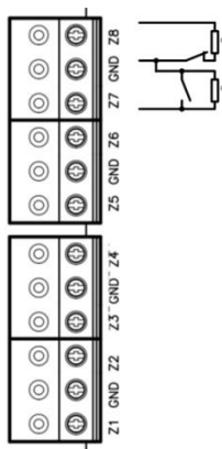
Рис.16. Подключение шлейфов блокировки и свободного прохода
