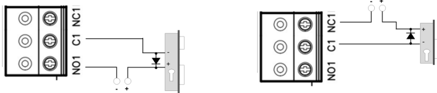
Рис.17. Подключение замков при использовании внешнего источника питания
