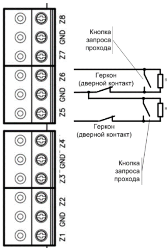
Рис.15. Подключение комбинированного шлейфа
