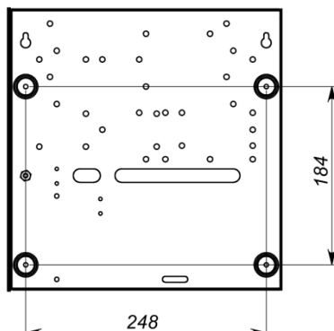
Рис 10. Разметка крепежных отверстий
