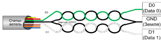
Рис.12. Подключение проводов data 0, data1 при использовании витой пары
