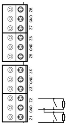
Рис.13. Подключение кнопки запроса прохода
