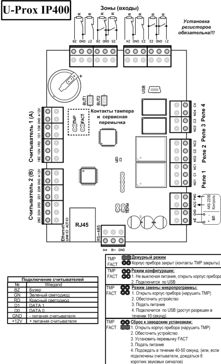
Рис. 2. Внешний вид платы контроллера
