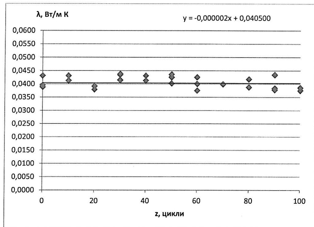
Рисунок 3 – Залежність теплопровідності виробів із мінеральної вати ТМ «ISOVER» марки «ISOVER Профи» від циклічних впливів
