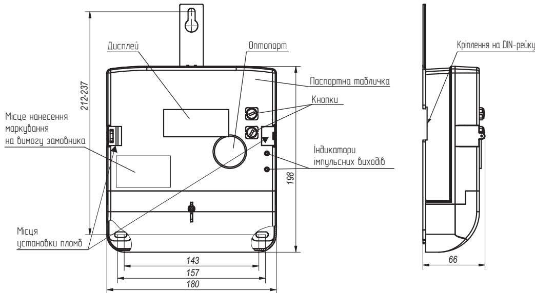
Малюнок А.1 - Загальний вигляд, габаритні і установчі розміри, місця установки пломб на корпусі трифазного лічильника трансформаторного включення типу МТХ 3G20...D.3...3-...4
