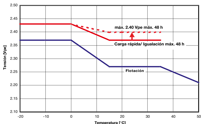
Fig. 3: A400/FT, A600, Powercycle; tensión de carga vs. temperatura
