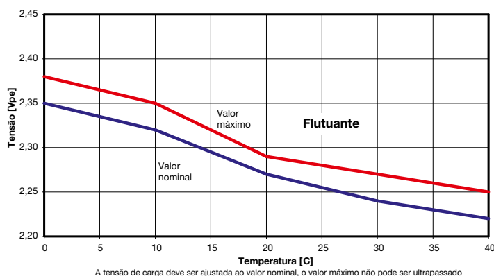
Fig.1: Marathon L/XL e Powerfit S100/S100L/S300; Tensão de carga vs. Temperatura
