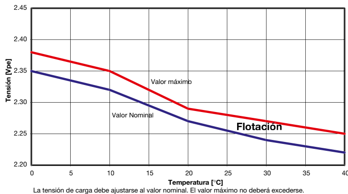
Fig. 1: Marathon L/XL y Powerfit S100/S100L/S300; tensión de carga vs. temperatura
