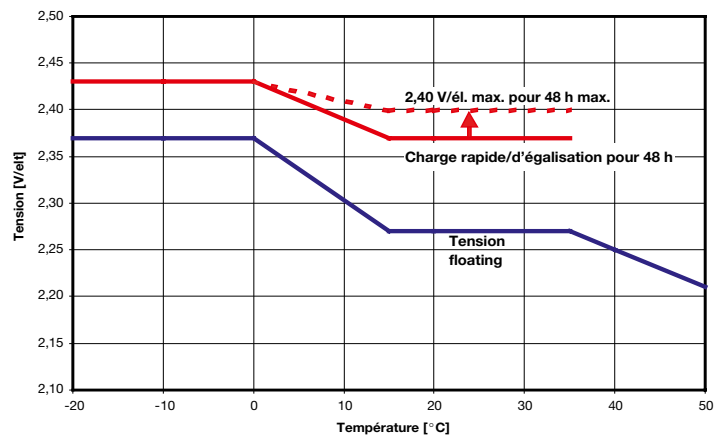
Figure 3: A400/FT, A600, Powercycle; tension de charge en fonction de la température
