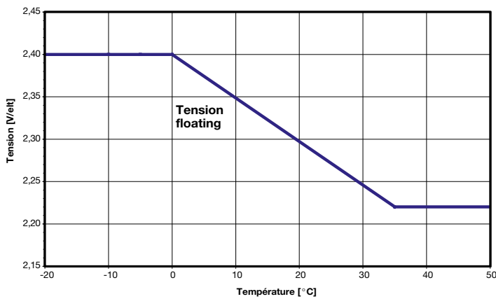
Figure 2: Marathon M-FT/FTX, Sprinter P/XP/FT; tension de charge en fonction de la température
