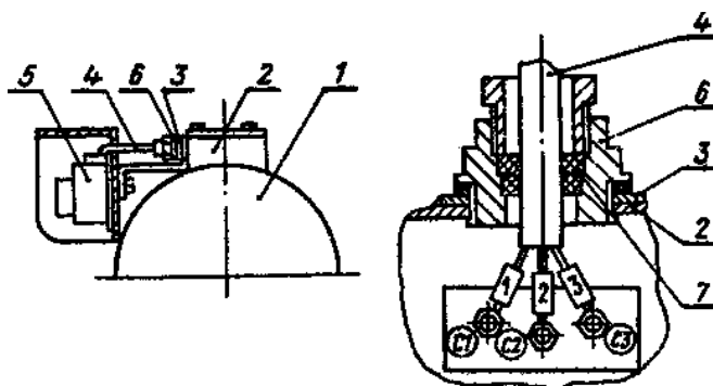
Рис. 5. К электродвигателю AIP100s2
