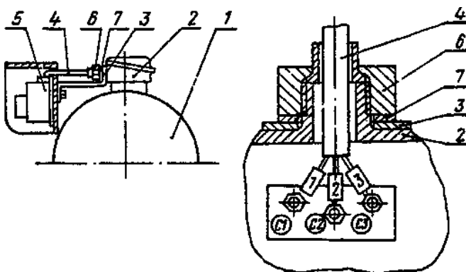
Рис. 6. К электродвигателю 4AM100s2
