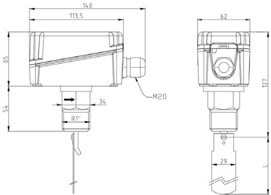
Dimensioner / Dimensions / Maßbild / Dimensions
