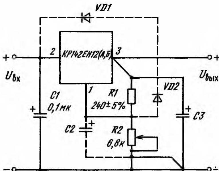
Типовая схема включения ИМС КР142ЕН12
