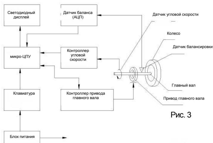
Рис. 3 Функциональная блок-схема балансирующего станка CB1930B
