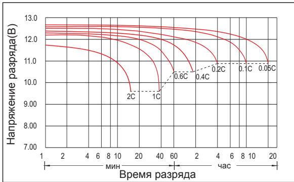
Характеристика разряда
