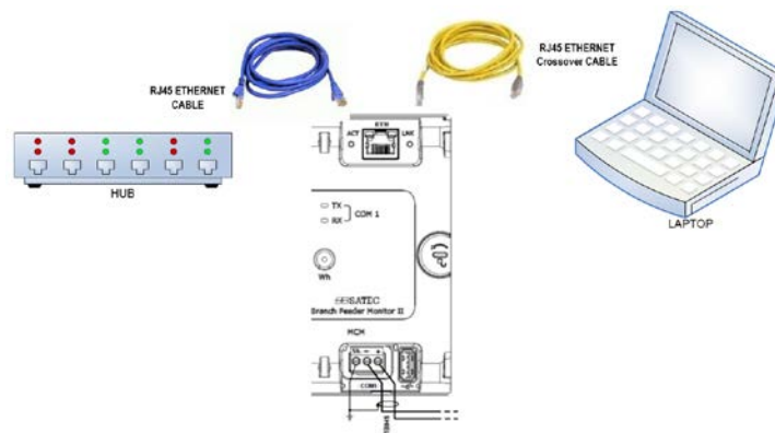
Рис. 19 Подключение прибора через порт ETH
