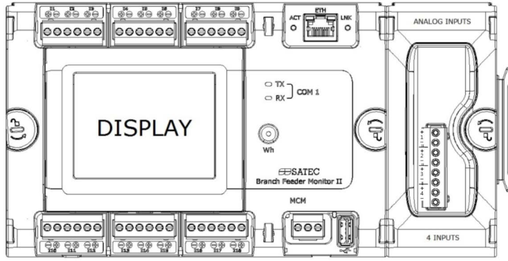
Рис. 14 Подключение модуля аналоговых входов к прибору
