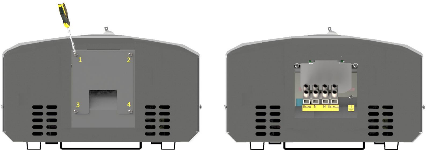
Рисунок 12. Схема снятия защитной крышки снизу корпуса стабилизатора
