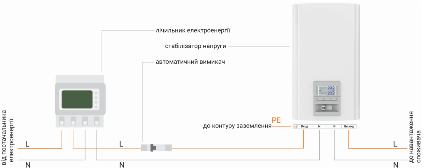
Рисунок 10. Схема підключення стабілізатора Герц і Герц-Дуо до однофазної мережі
