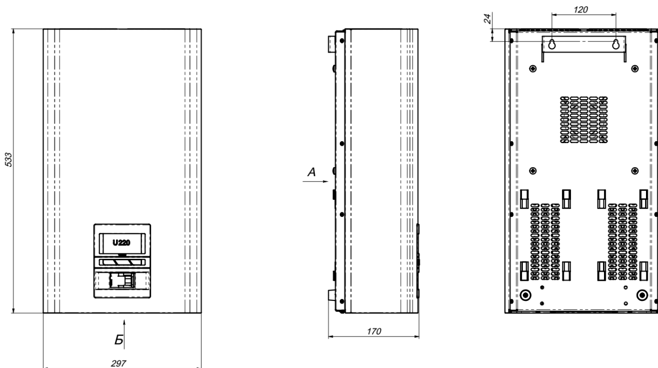
Рисунок 8. Установчі та посадочні розміри стабілізаторів Герц і Герц-Дуо на 50-63-80А
