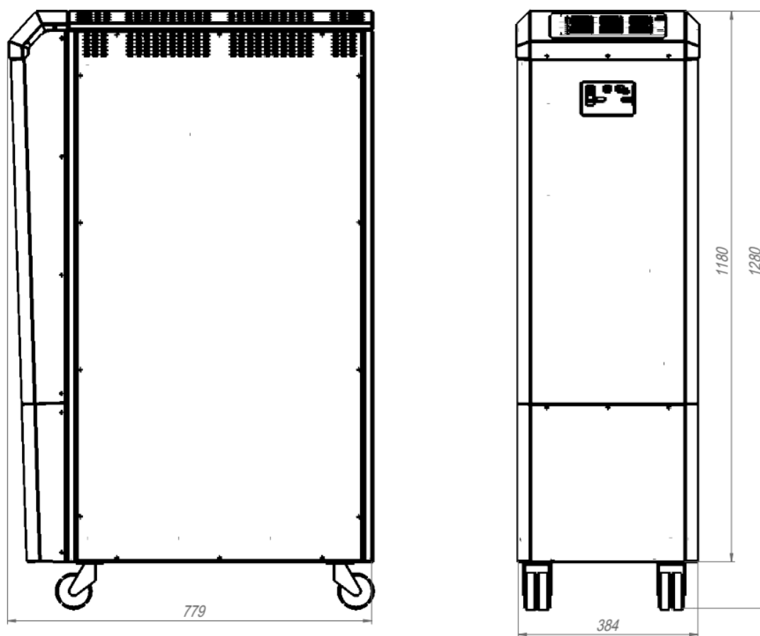
Рисунок 9. Габаритні розміри стабілізатора Герц-ПРО на 100-160А
