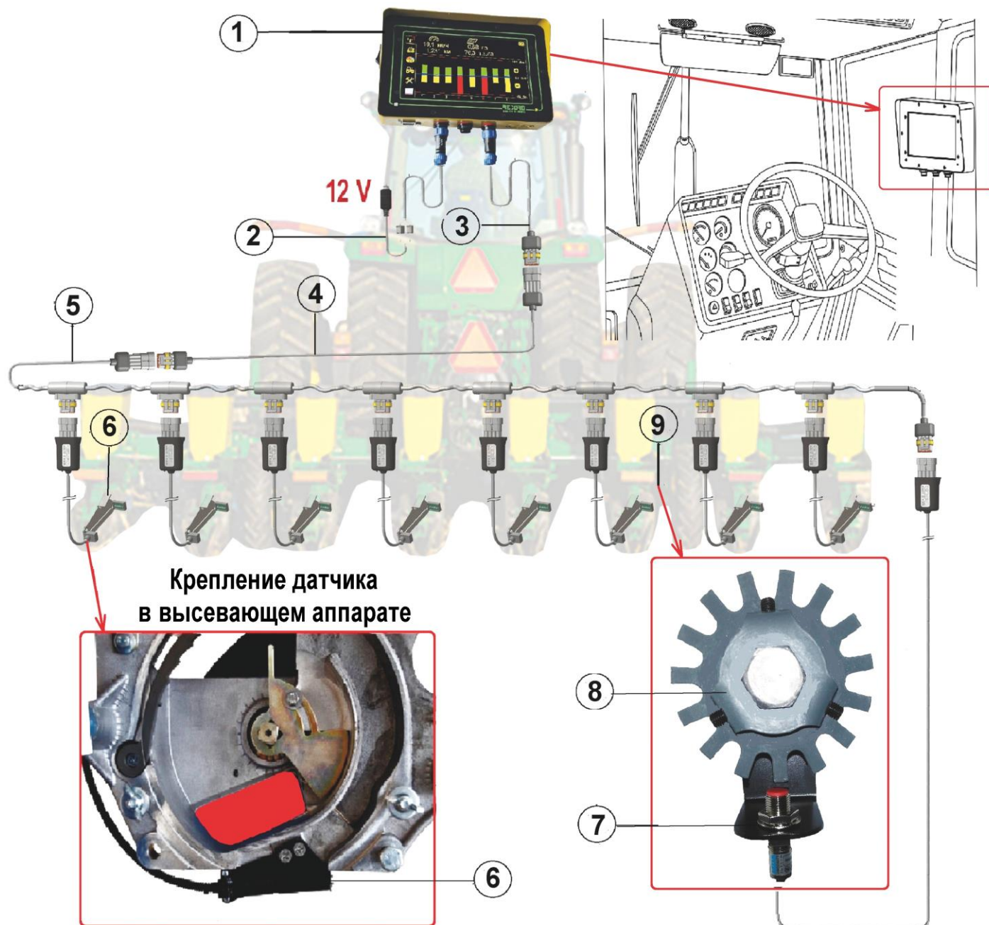
Схема размещения СКВ «Record» на технике рис.1
