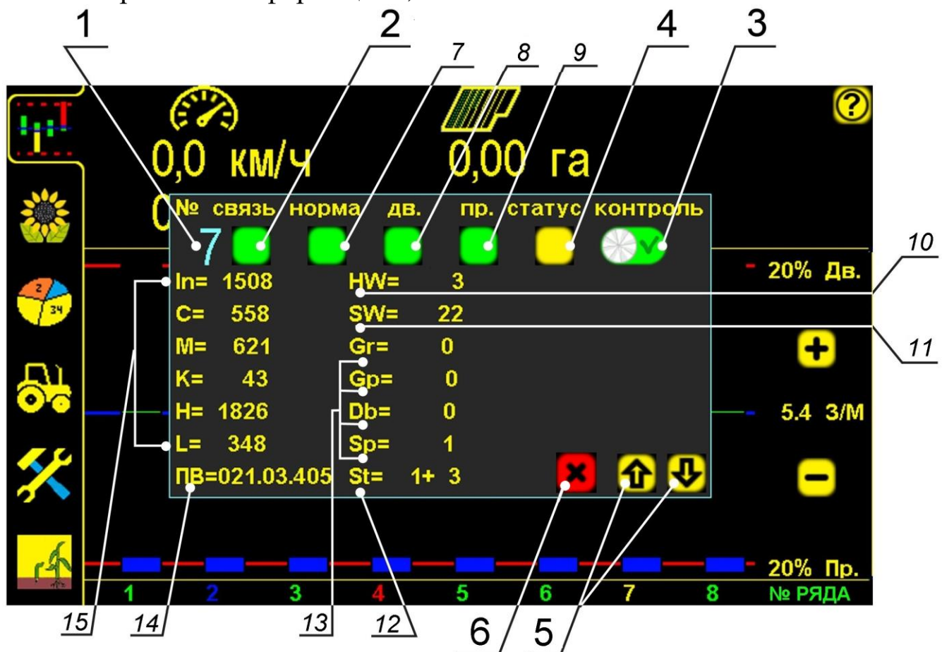
«Окно показателей датчика высева» рис.36
