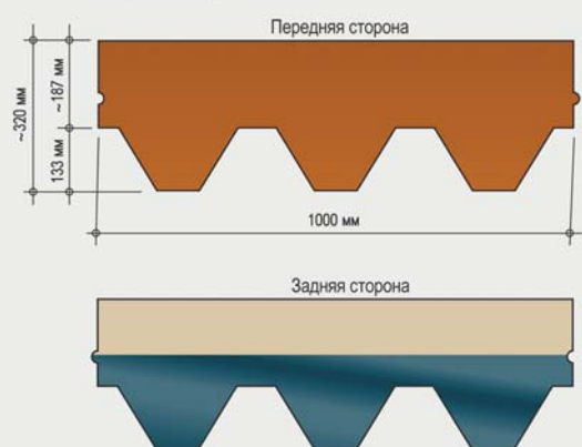
Размеры Jazzy, KL, Katrilli
