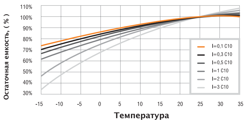
Емкостно-температурная зависимость
