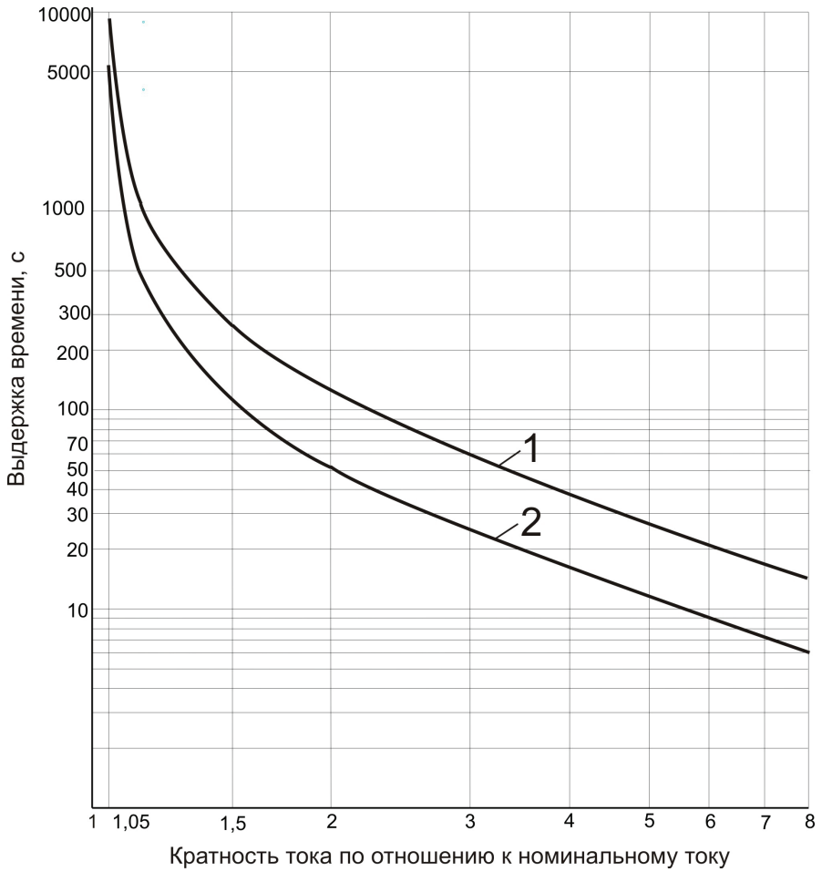
Рис. 2.1 Номинальные время-токовые характеристики реле РЭЗЭ-6М :
