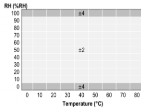
Мал. 1. Похибка вимірювань
