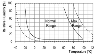
Мал. 2. Умови експлуатації
