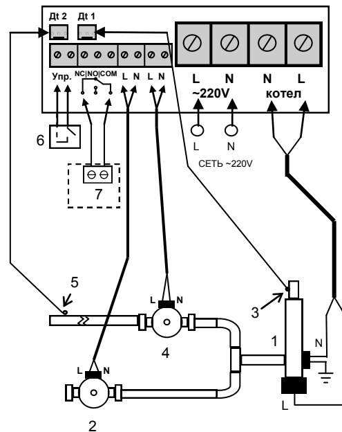
Рис.2. Подключение проводов питания, нагрузки, управления и датчиков температуры при работе на две системы циркуляции теплоносителя (с двумя цифровыми датчиками температуры).
