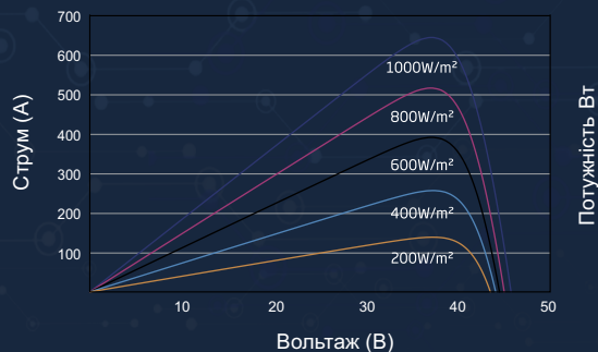
Крива струму та напруги
