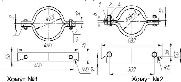
1 – Скоба; 2 – Гайка М 16; 3 – Болт М 16x40; 4 – Болт М 16x70 Рисунок 3. Монтажные хомуты.
