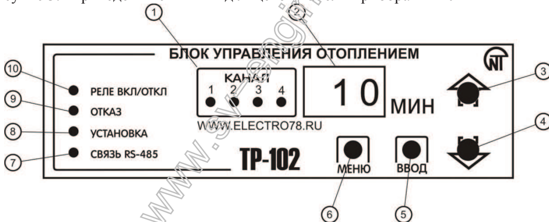
Рисунок 3.2 – лицевая панель TP-102
