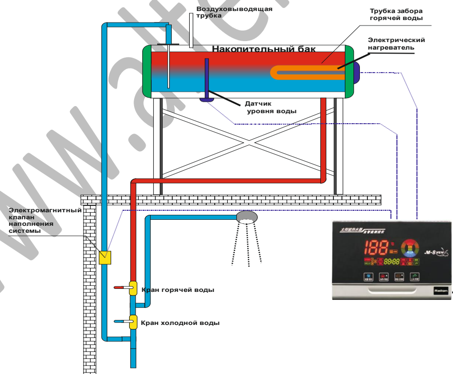
Рис. 2.3 Схема безнапорной системы с электронным наполнением бака
