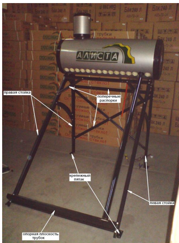
Рис. 2.5 Общий вид в сборе рамы солнечной системы нагрева воды
