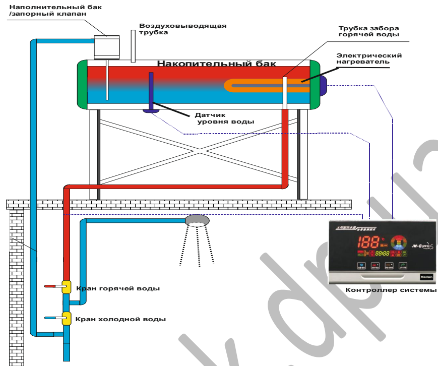
Рис. 2.2 Схема безнапорной системы с механическим наполнением бака
