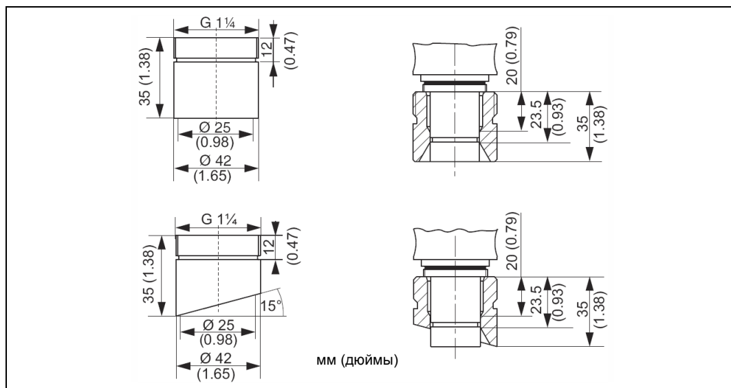
Приварные фитинги
