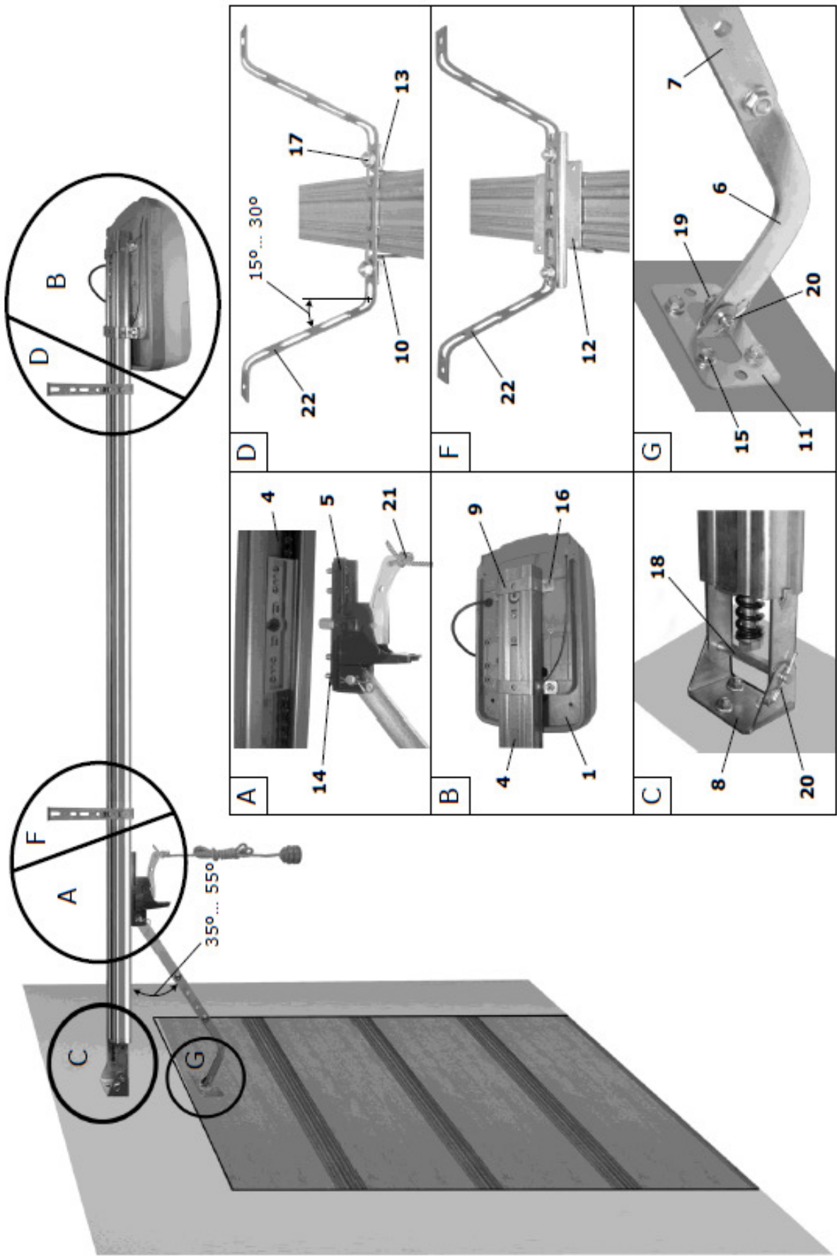
Рис. 2. Монтаж комплекта
