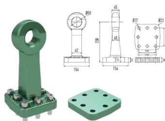
Закордонний кронштейн дишла
