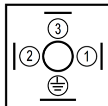
DIN 43650-C SOCKET
