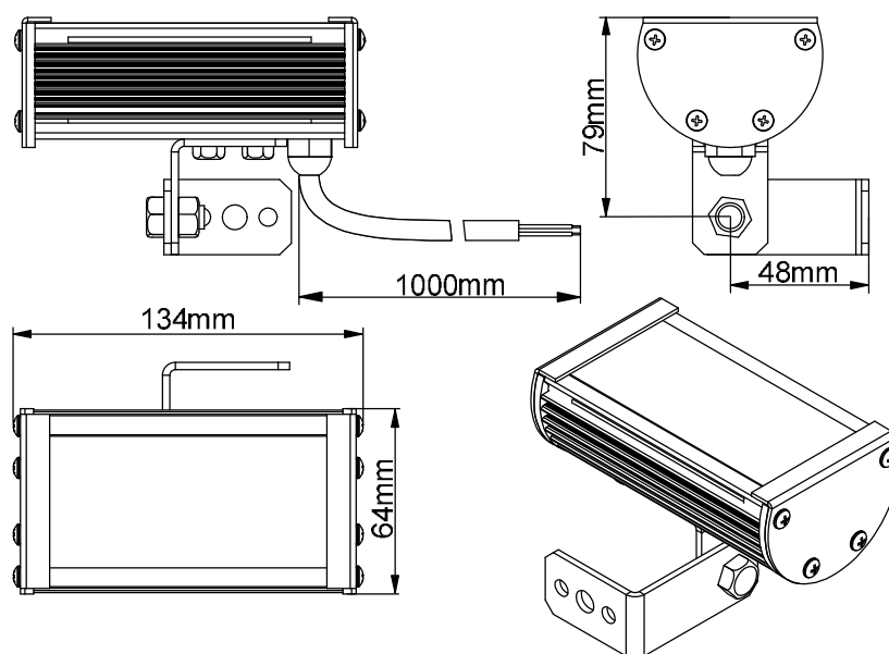
Габаритные размеры светильника LS Line-1-XX-02-24V
