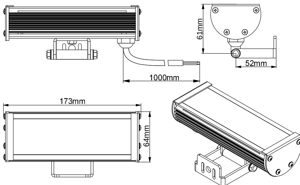
Габаритные размеры светильника LS Line-1-XX-03-24V
