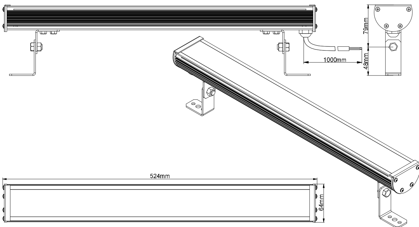
Габаритные размеры светильника LS Line-1-XX-12-24V
