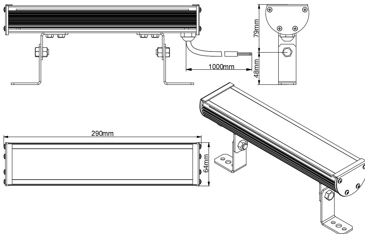
Габаритные размеры светильника LS Line-1-XX-06-24V
