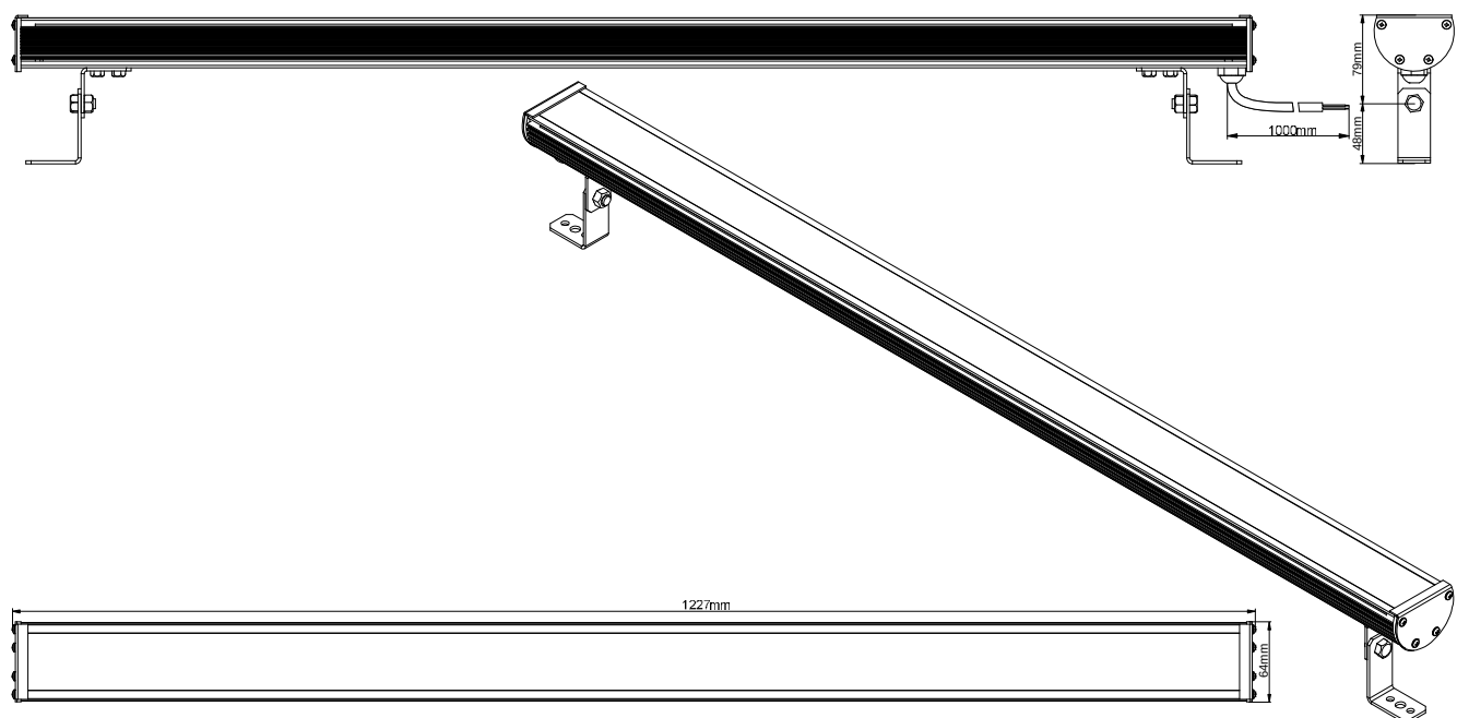
Габаритные размеры светильника LS Line-1-XX-30-24V
