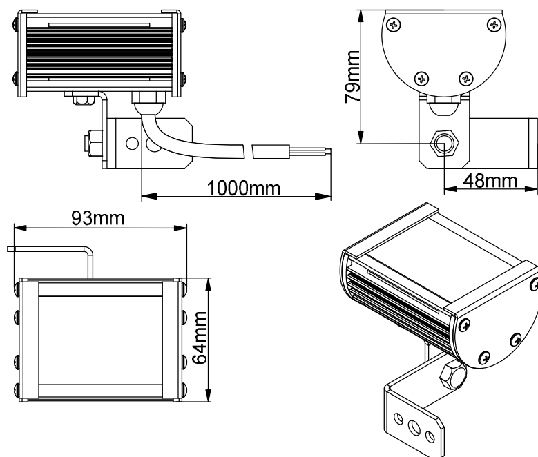
Габаритные размеры светильника LS Line-1-XX-01-24V
