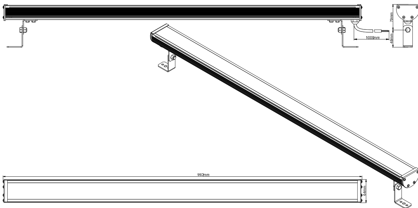
Габаритные размеры светильника LS Line-1-XX-24-24V
