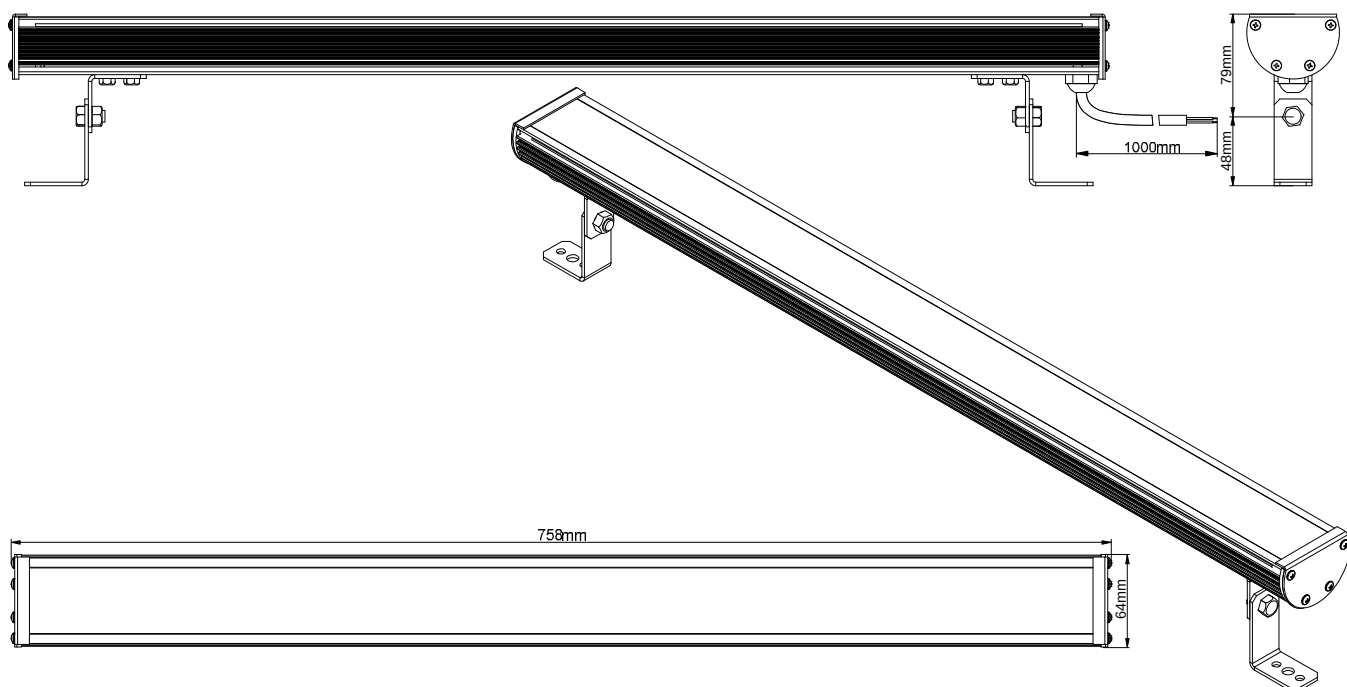
Габаритные размеры светильника LS Line-1-XX-18-24V
