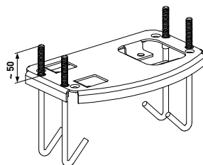
Рисунок 3. Монтажное основание
