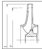
Reduction du diamètre extérieur de la roue pour pompe centrifuge par tournage.
