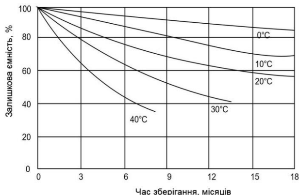
Мал. 1. Характеристики саморозряду акумулятора
