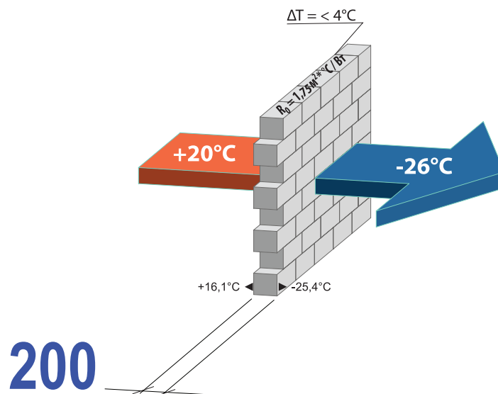
Мал. 1.1. Стіна з газобетону D400 товщиною 200 мм забезпечує тепловий комфорт
