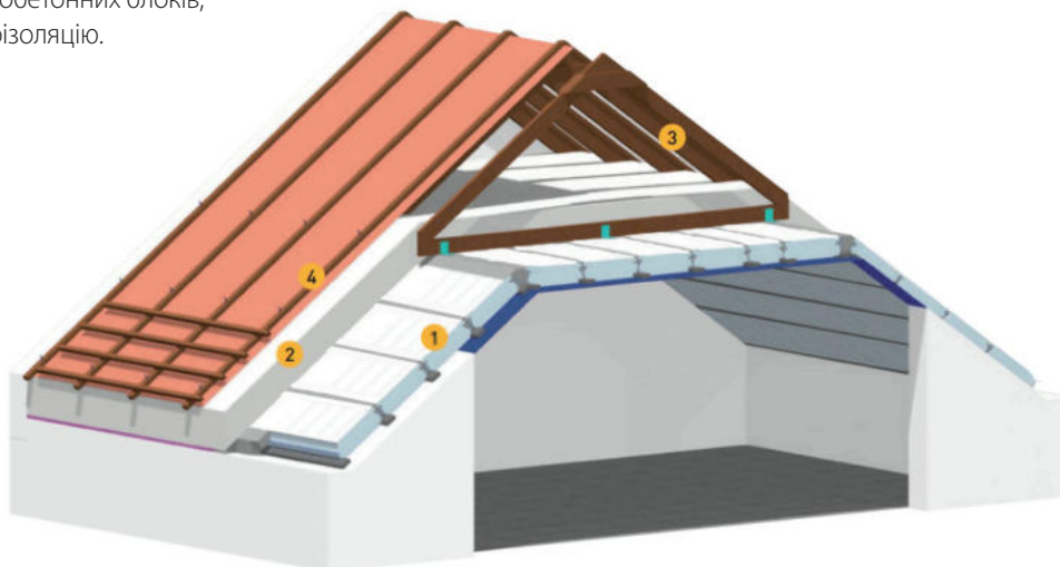
Мал. 7.18 Система ізоляції скатної покрівлі AEROC Energy
