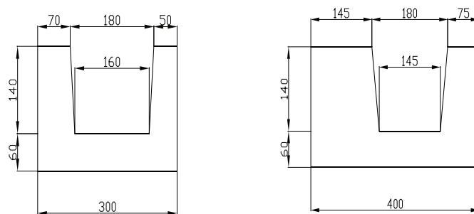
Мал. 5.2 U-блоки AEROC
