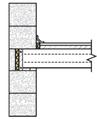
г) перекриття збірне із залізобетонних плит
