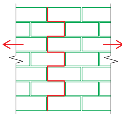
Мал. 3.2 Розтяг кладки по перев'язаному перетину
