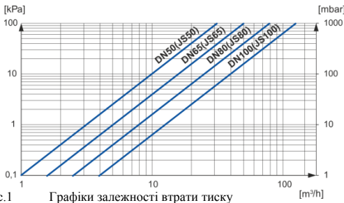
Рис.1 Графіки залежності втрати тиску лічильників від об'єму витрати
