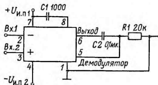
Функциональная схема включения ИМС 140УД13, К140УД13
