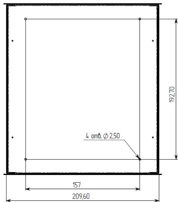
СЕЧЕНИЕ А-А
