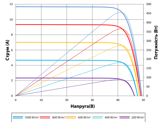
Крива струму та напруги (455S)
