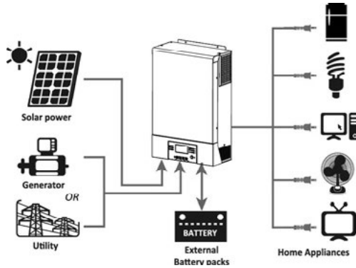
Малюнок 1 Основний тип фотоелектричної системи
