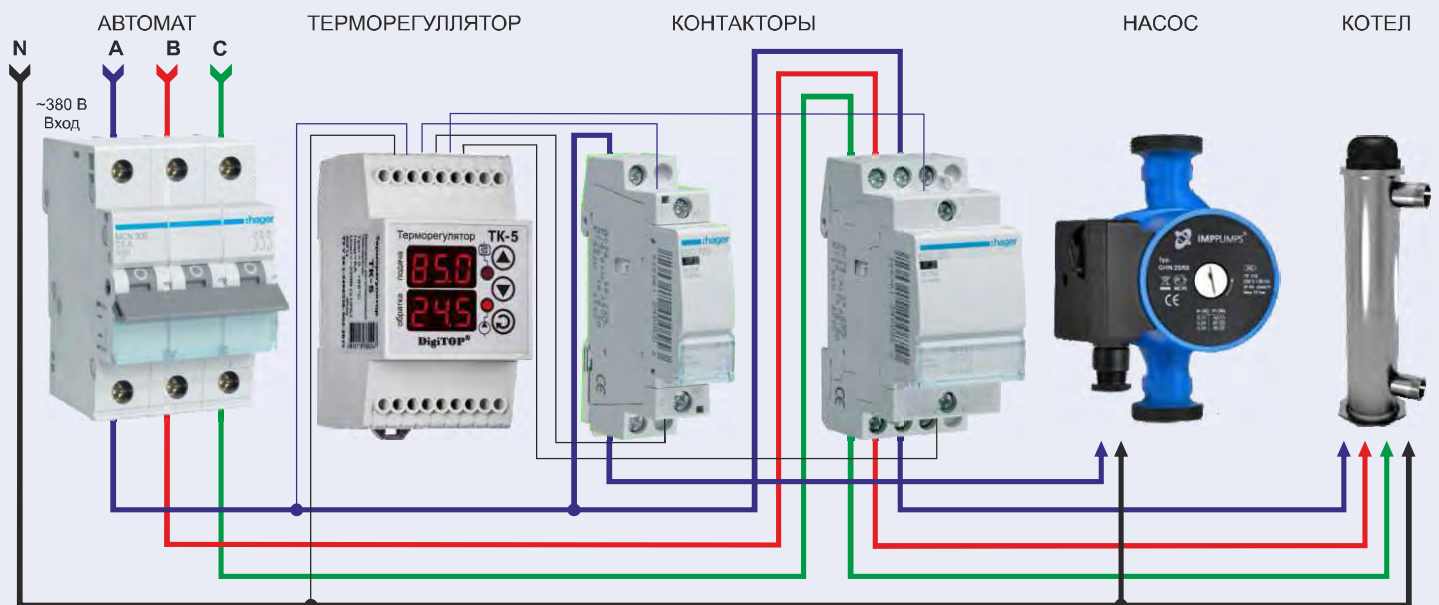
Пример комплектации блока управления трехфазным электрическим котлом и однофазным насосом с использованием терморегулятора ТК-5 / ТК-5а
