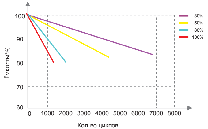
Влияние глубины разряда на срок службы
