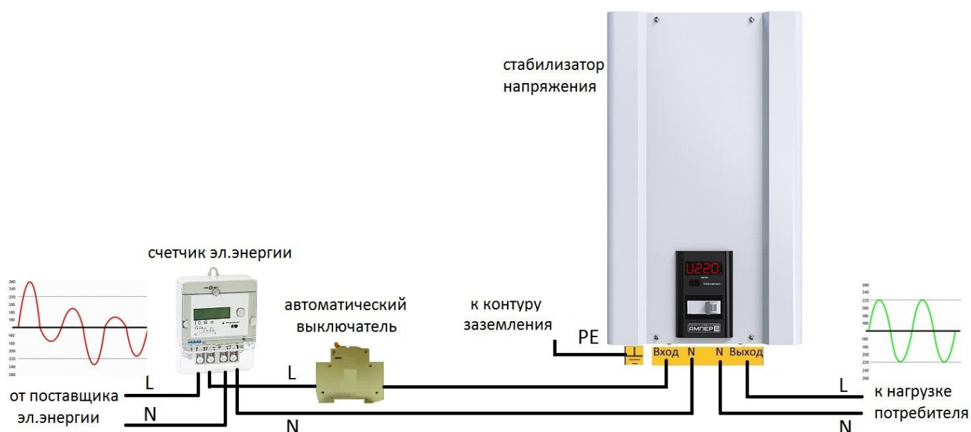
Рисунок 11. Схема подключения стабилизатора к однофазной сети
