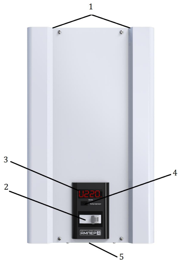
Рис.1 Зовнішній вигляд стабілізатора АМПЕР на 25-80А
