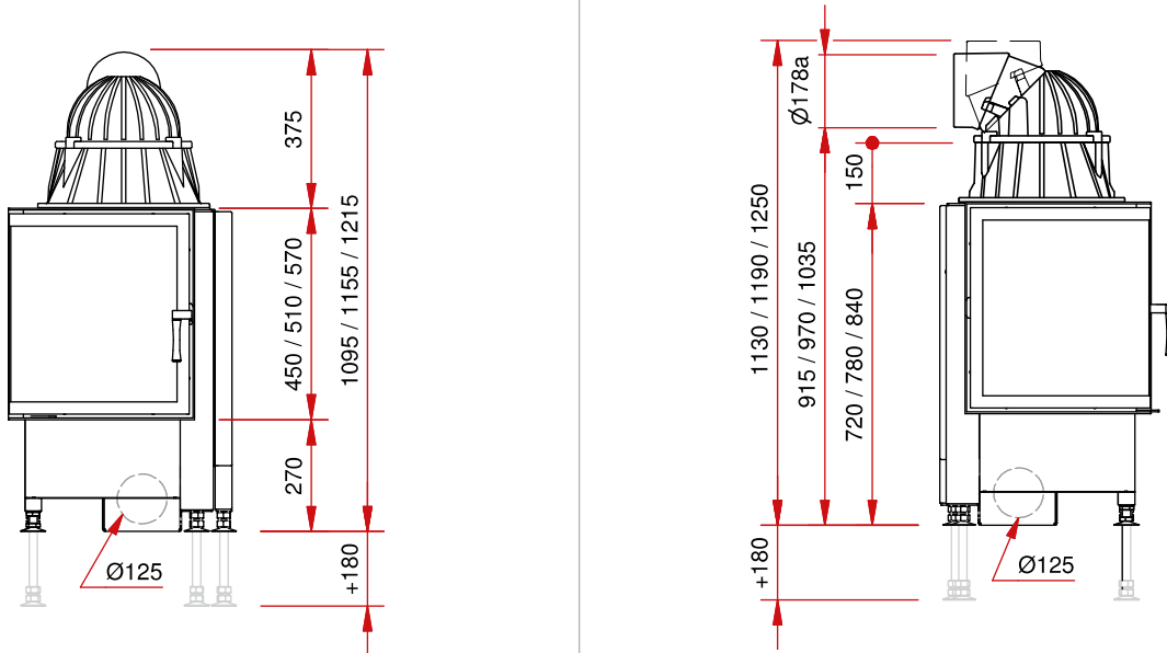
Изображение сверху М 1:10
