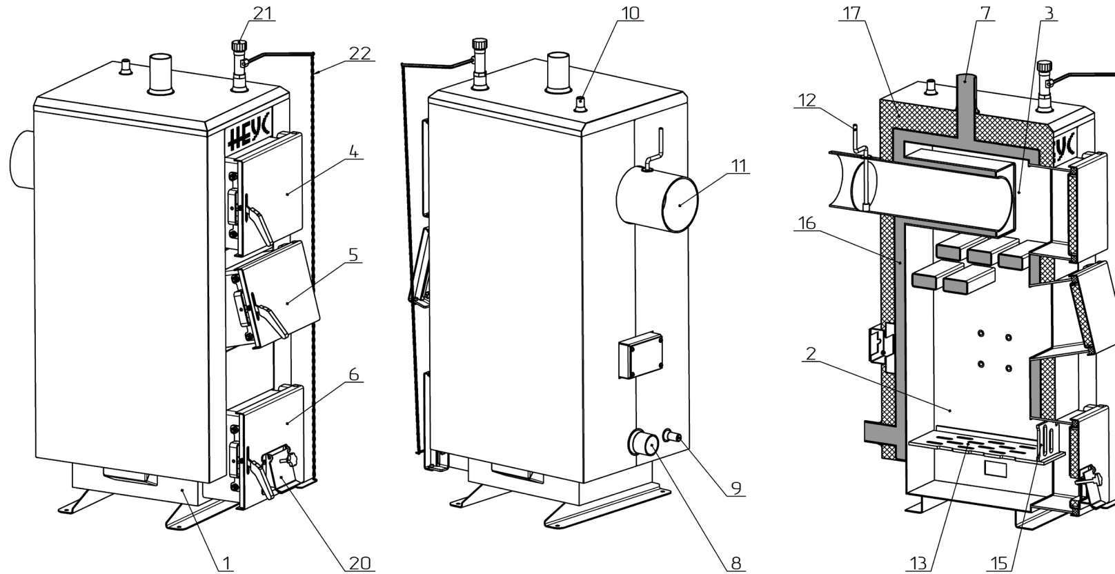
Рисунок 2б – Основні елементи котла Неус-КТМ
