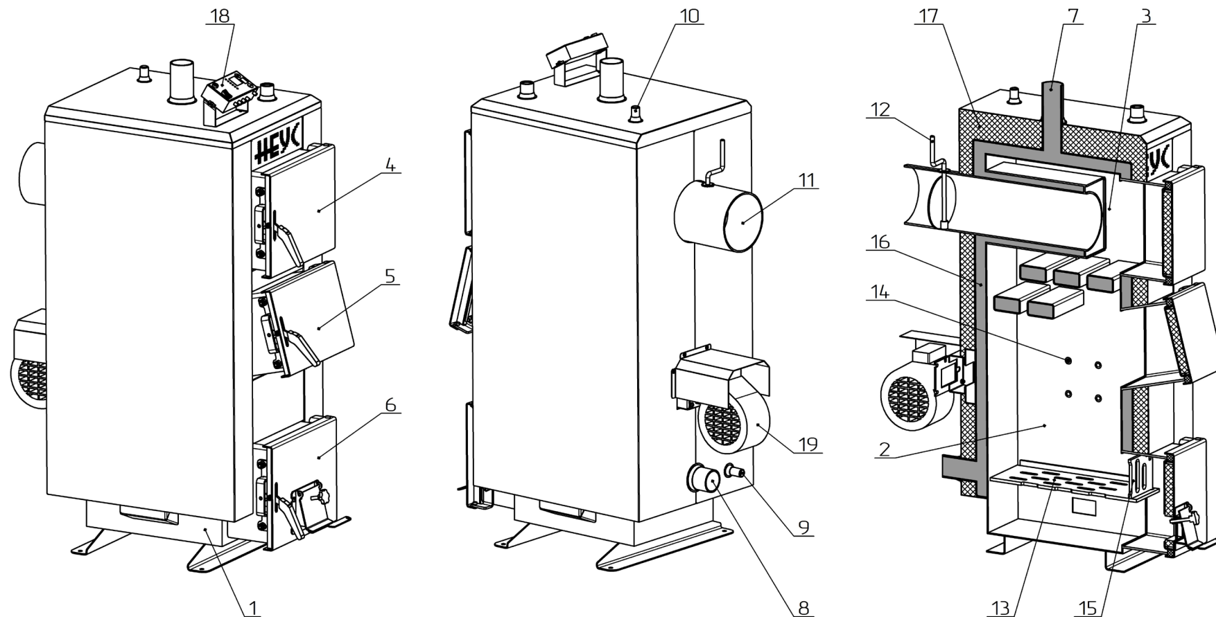
Рисунок 2а – Основні елементи котла Неус-КТА
