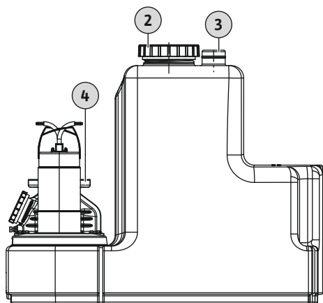
Fig. 6: Під'єднання припливно-витяжної вентиляції до збірного резервуару
