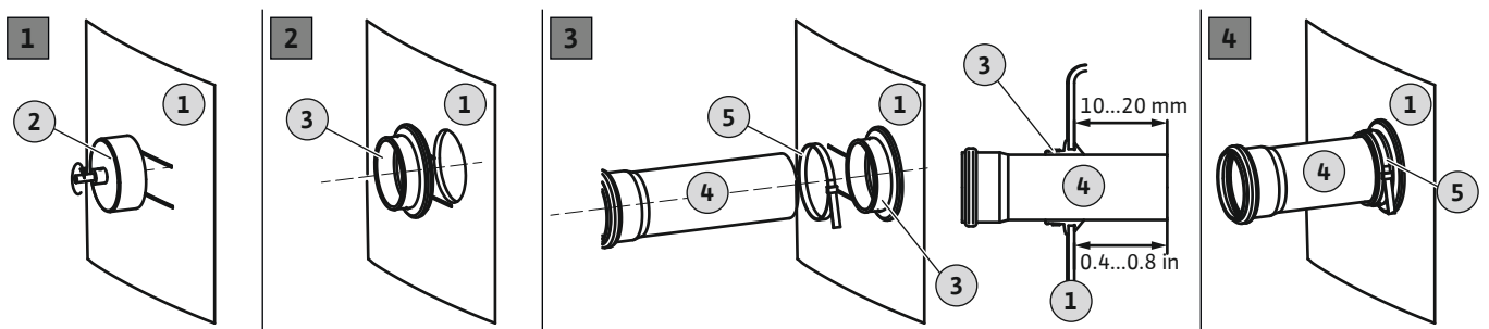
Fig. 5: Під'єднання приточного трубопроводу
