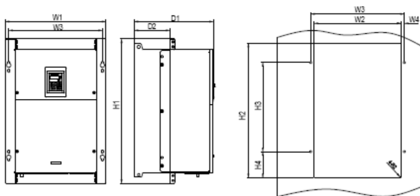
Фланцевое крепление инверторов 3 ф. 380 В мощностью 90~110 кВт
