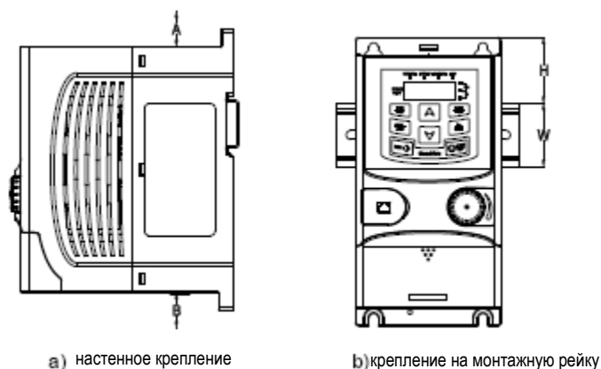
Рис. 3-1: Установка инвертора
