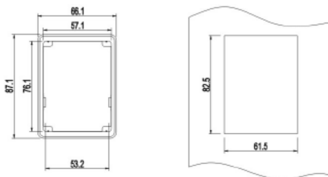
Монтажный кронштейн
