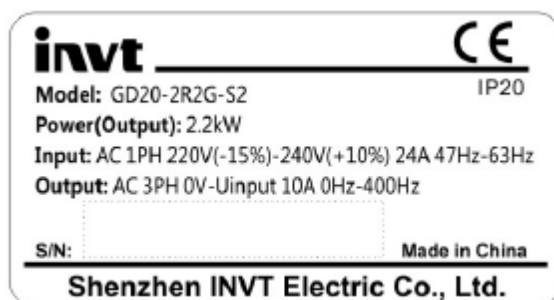
Рис. 2-1: Заводская табличка
