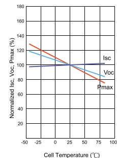
Залежність температури від I_{sc} , V_{oc} , P_{max}
