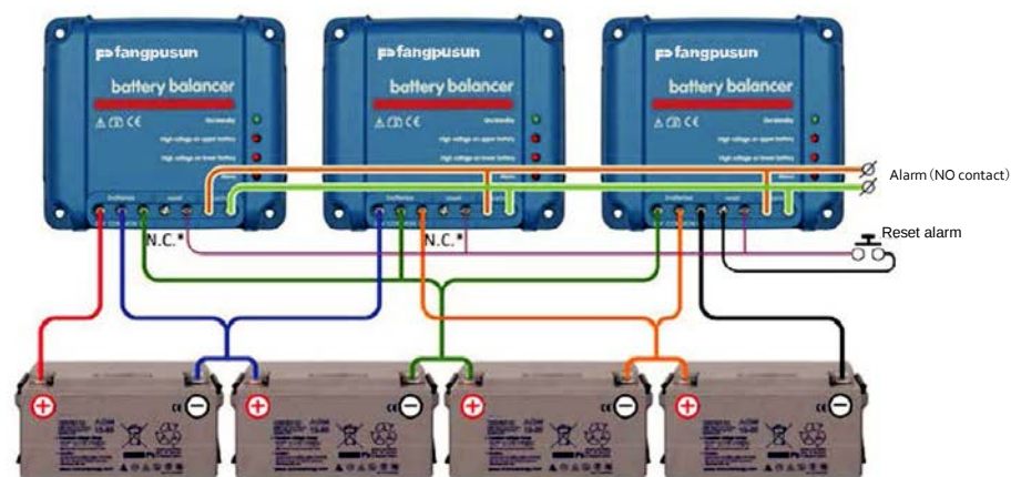
Три акумуляторні балансири підключені до чотирьох послідовно з'єднаних батарей 12В (система 48В)
