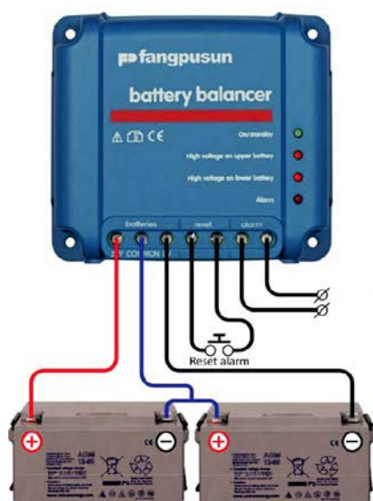
Балансир акумулятора, підключений до двох послідовно з'єднаних батарей 12В (система 24В)
